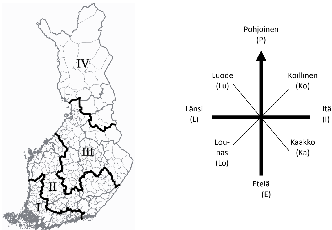
Kuva L1.1. Säävyöhykkeet ja ilmansuuntien lyhenteet.
